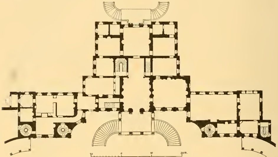
Fig. 150. Hopetounhouse. Grundriss.
